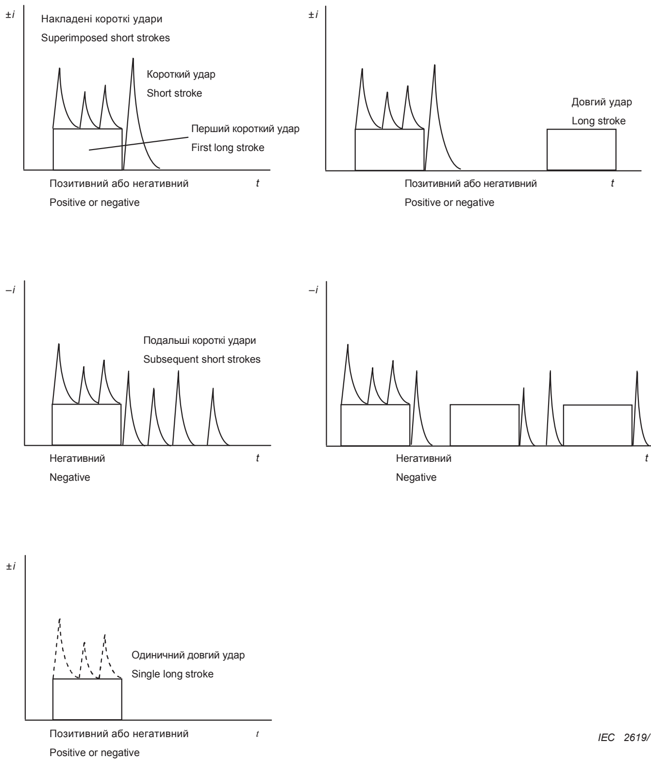
Рисунок А.4 - Можливі компоненти верхобіжних спалахів (характерні для будівель (споруд), що витикаються на місцевості або панують над оточенням)
